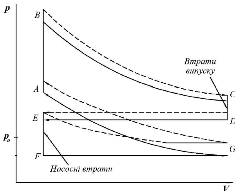
Рис. 2 Індикаторні діаграми ДВЗ при звичайному (—) і пропонуваному (---) способах роботи
