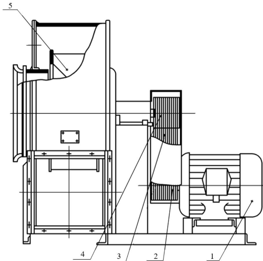
1 – електродвигун; 2 – тяговий шків; 3 – пасова передача; 4 – ведений шків; 5 – колесо вентилятора
