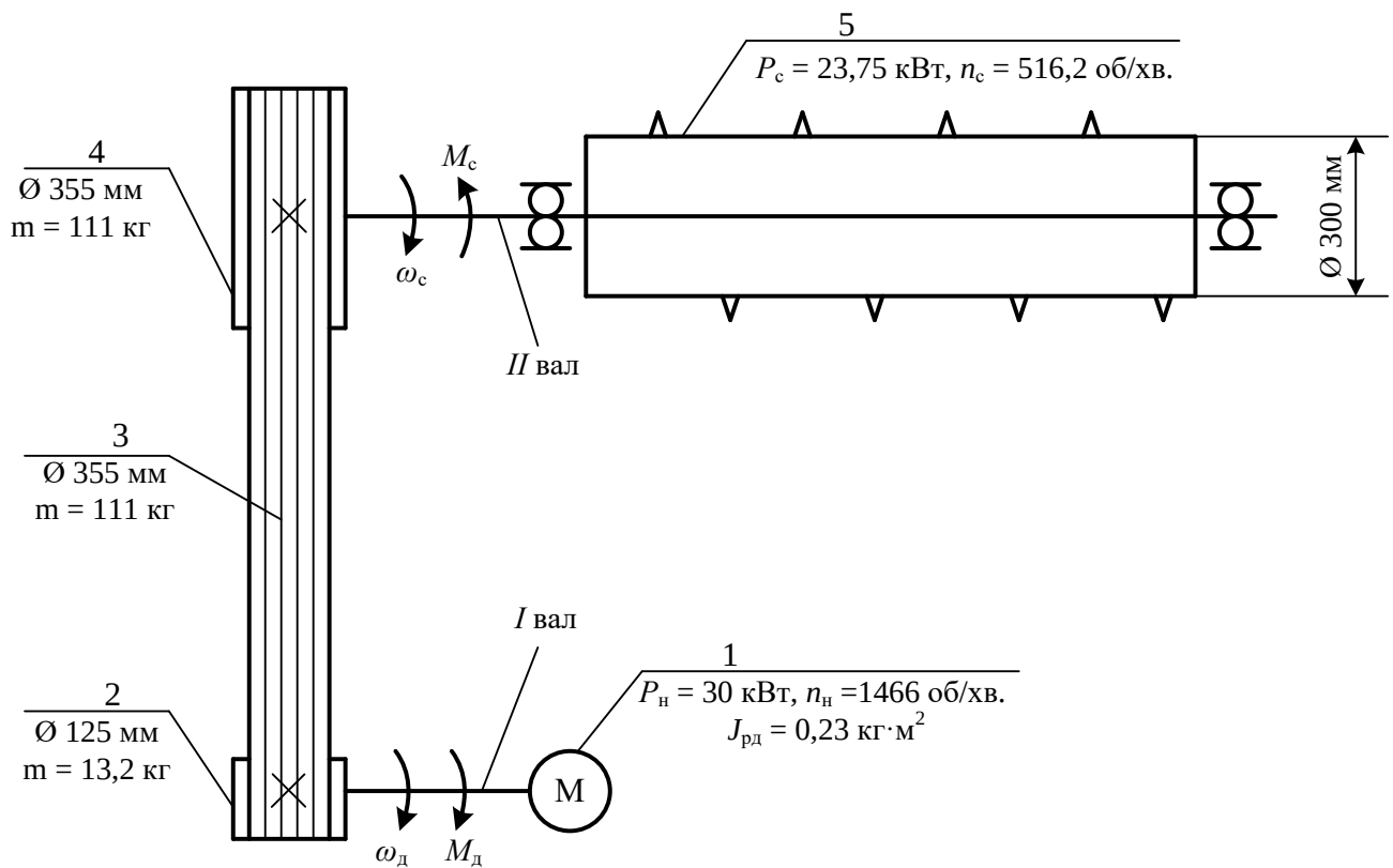
Рисунок 5 – Зразок кінематичної схеми вентилятора
