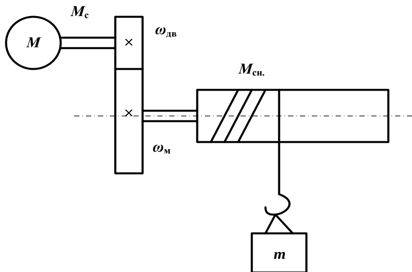
Рисунок 2 – Кінематична схема з ланкою, що рухається поступально
