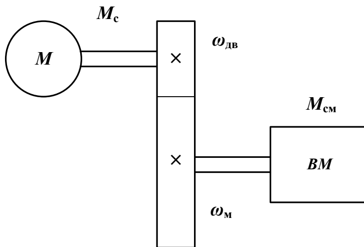
Рисунок 1 – Кінематична схема з обертовим виконавчим механізмом
