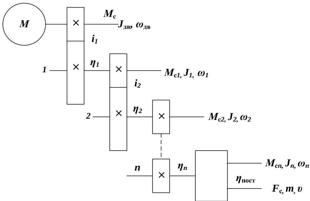
Рисунок 3 – Кінематична схема багатоланкової системи
