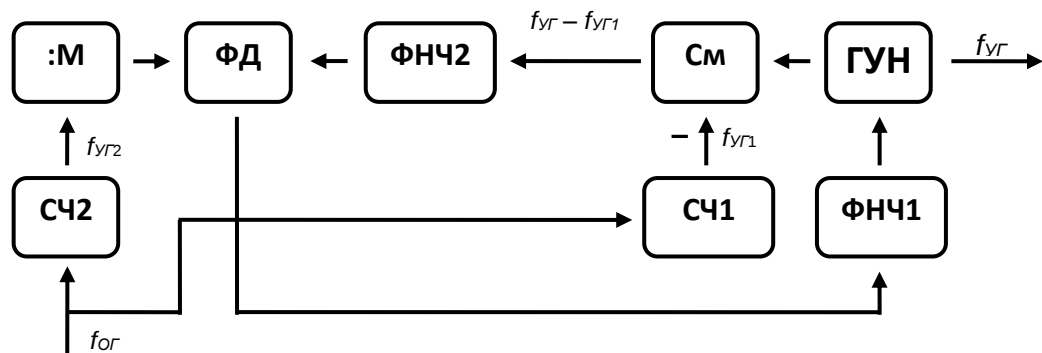
Рисунок 4 - Структурная схема трехкольцевого синтезатора частоты
