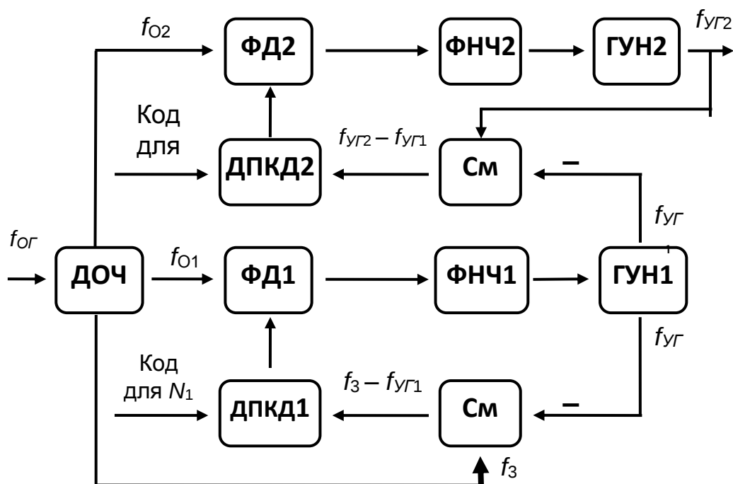
Рисунок 3 - Структурная схема двухкольцевого синтезатора частоты
