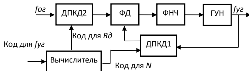
Рисунок 2 - Структурная схема синтезатора с аппроксимацией значений выходных частот
