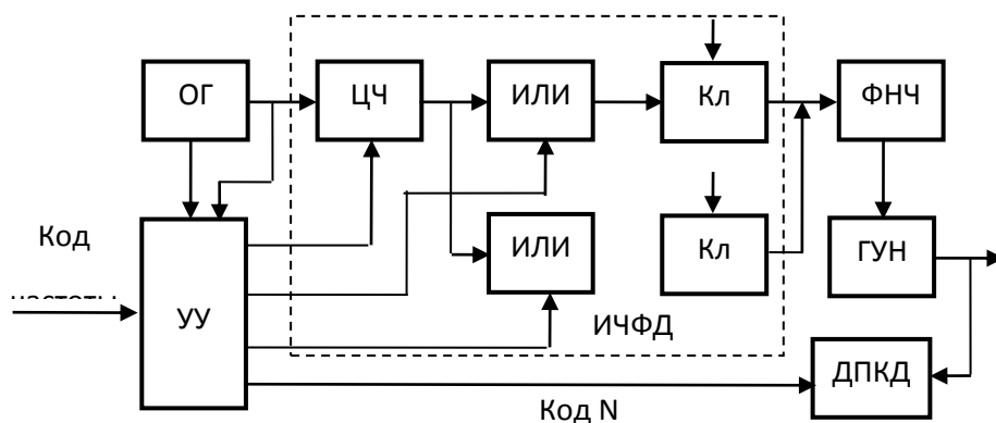
Рисунок 1 - Структурная схема СЧ с ИЧФД
