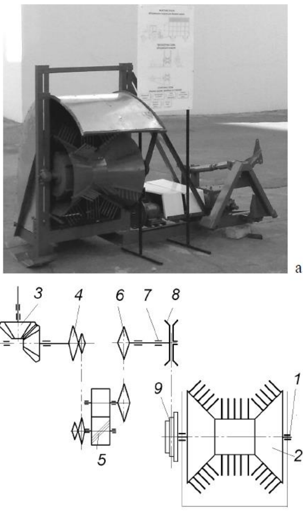
Рис. 4. Загальний вид (а) і кінематична схема (б) очісувального модулю: 1 - рама; 2 - очісувальний барабан; 3 – конічний редуктор (передаточне відношення 1:1); 4 – ланцюгова передача; 5 – циліндричний одноступеневий редуктор (передаточне відношення 1:1); 6 – ланцюгова передача; 7 – опора підшипникова проміжна; 8 – варіатор механічний; 9 – пасова передача.
