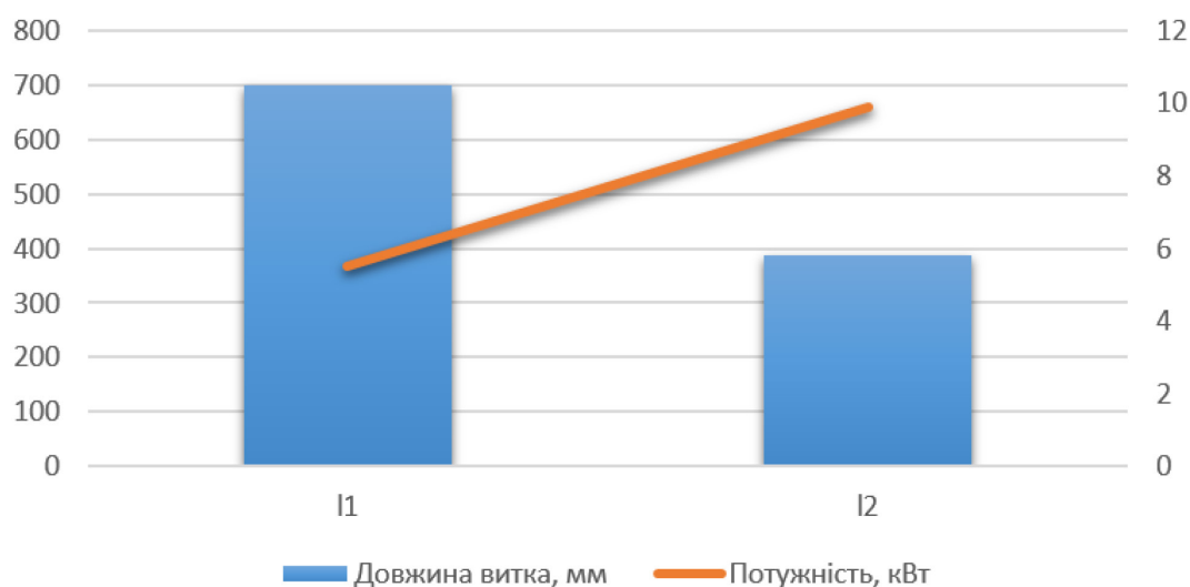
Рис. 4. Діаграма зміни потужності залежно від зміни довжини витка обмотки.
