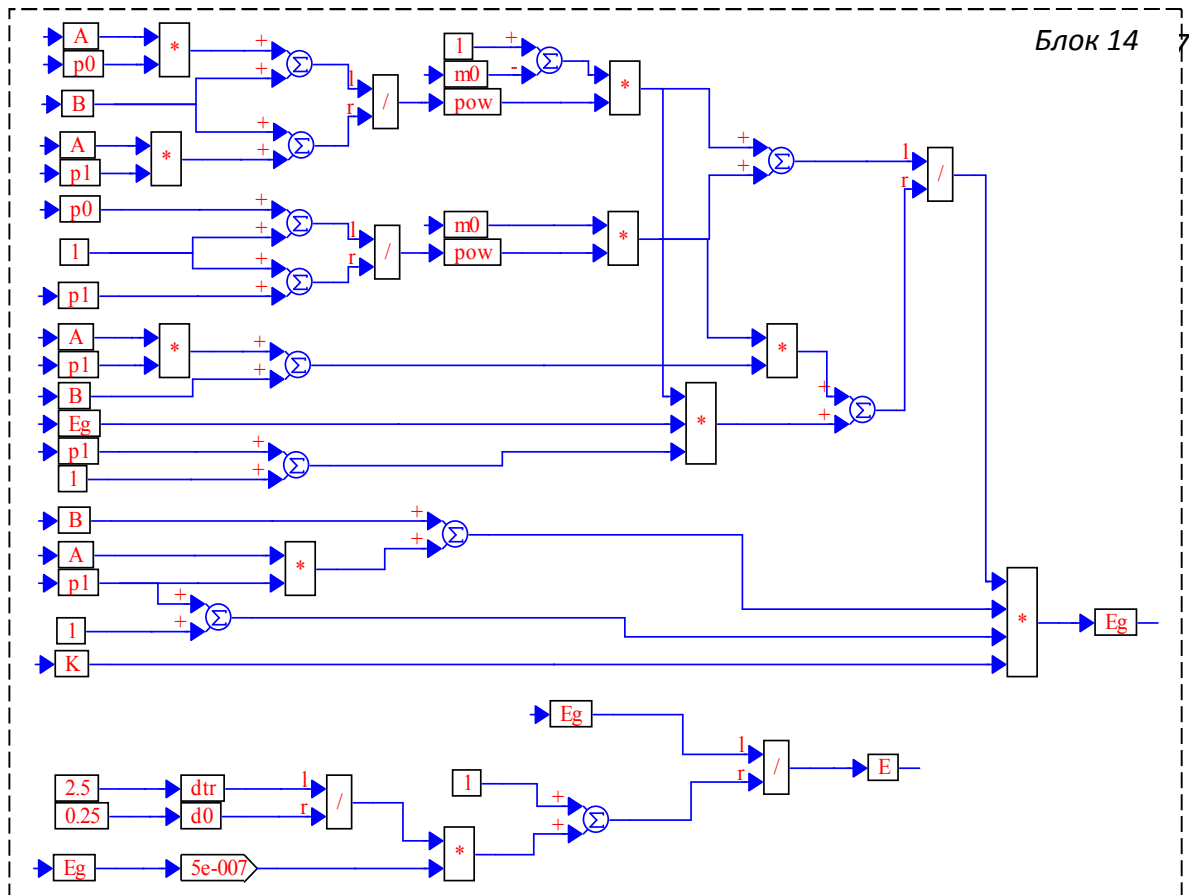
Рис. 14. Блок моделювання двофазної робочої рідини
