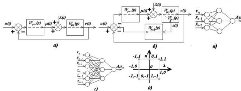
Рис. 1. Схеми систем автоматичного керування, що досліджувалися: а – одноконтурна САК; б – САК з ПІ-регулятором і диференціатором; в, г – нейрорегулятор, відповідно, з трьома і шістьма входами; д – повна репліка комбінацій збурень \lambda(t) і u(t)
