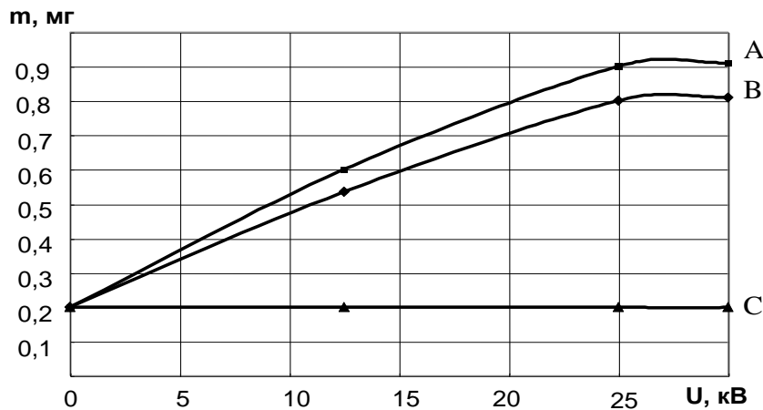
Рис. 1. Залежність маси зразка від напруги блока живлення
