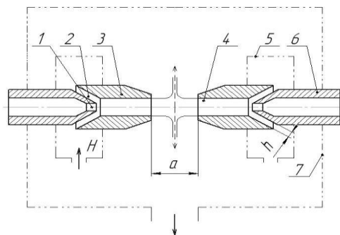
Рис. 1. Схema протитечію-струминного змішувача: 1 – робоче сопло; 2 – камера ежекції; 3 – камера змішування; 4 – сопло камери змішування; 5 – камера подачі підмішуваного компонента; 6 – робочий патрубок; 7 – камера збирання рідини; а – відстань між соплами; Н – напір подачі підмішуваного компонента; h – кільцевий зазор камери ежекції
