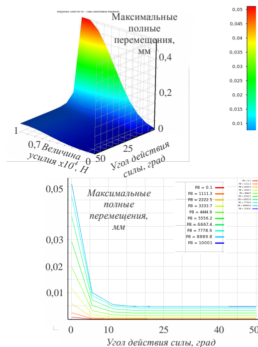
Рис. 19 – Зависимость полных перемещений верхнего среза колонки от параметров p_1, p_2 (задача 2.1)
