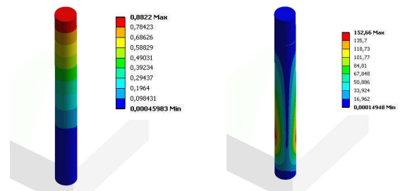
Рис. 17 – Распределение полных перемещений в колонке штампа (задача 2.1)
