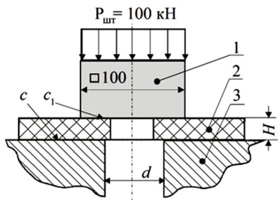
Рис. 3. Расчетная схема нижней плиты во взаимодействии с пакетом и подштамповой плитой пресса [3]:
