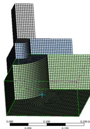
Рис. 4. Конечно-элементная модель нижней плиты во взаимодействии с пакетом и подштамповой плитой пресса
