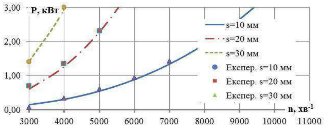
Рис. 1. Графік залежності експериментальної потужності ПГ P від частоти n і амплітуди r коливань поршня та порівняння її з теоретичними даними для конічних отворів поршня
