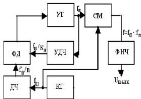
Рисунок 2 – Возможная схем косвенного синтеза частот
