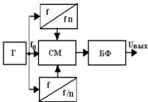
Рисунок 1 – Возможная схема прямого метода синтеза
