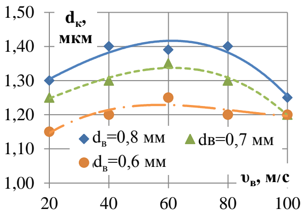
Рис. 17. Залежність середнього діаметра жирових кульок d_k від швидкості v_в і діаметра каналу подачі молочних вершків d_в СГРЖФ (при v_{зп} = 60 м/с)
