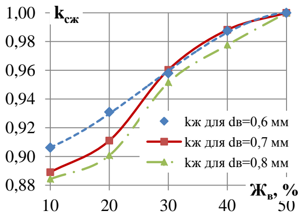
Рис. 19. Залежність коефіцієнта жирності вершків для СГРЖФ k_{сж} від жирності вершків J_в , при v_{зн}=80 м/с
