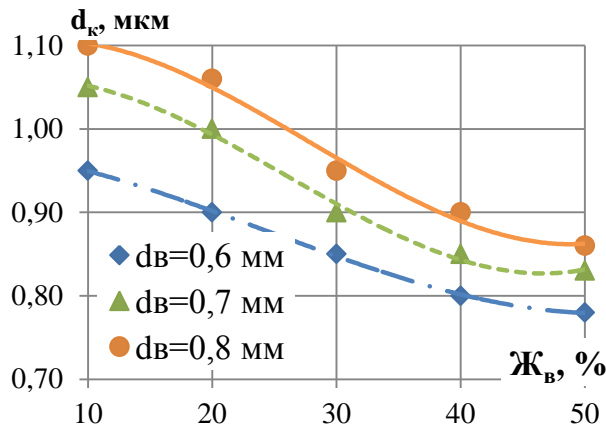
Рис. 18. Залежність середнього діаметра жирових кульок d_k від діаметра каналу подачі вершків d_e СГРЖФ та жирності вершків J_в (при v_{зн}=80 м/с)
