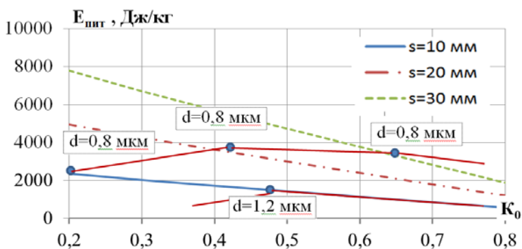
Рис. 13. Графік залежності питомих енерговитрат E_{num} від коефіцієнта живого перетину K_0 і амплітуди коливання поршня s ( D=60\text{мм} , \varphi=0,5 , n=3000\text{хв}^{-1} , K_2=100 )
