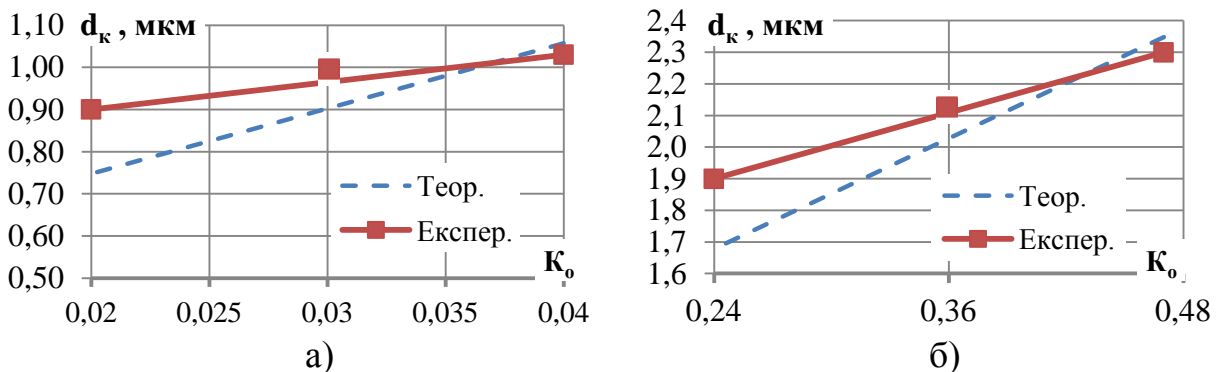
Рис. 24. Залежність середнього діаметра жирових кульок d_k від коефіцієнта живого перетину поршня K_o : а) – конічні отвори при n=6000 \text{ хв}^{-1} , s=10 \text{ мм} ; б) – циліндричні отвори при n=9000 \text{ хв}^{-1} , s=10 \text{ мм}
