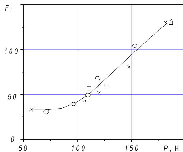
Рис. 2. Залежність між показниками, отриманими на приладах Фрайтестер та ДА-2М для шліфпорошку алмазу зернистістю 315/250:
