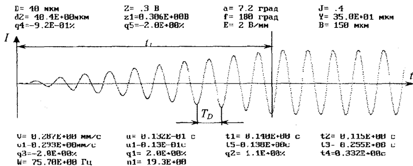
Рис. 5 – Вид доплеровского сигнала, полученного в результате теоретического расчета на ПЭВМ: D = 40 \text{ мкм} ; \xi = 0,3 \text{ В} ; \alpha = 7,2^\circ ; d = 150 \text{ мкм} ; V = 0,287 \text{ мм/с} .
