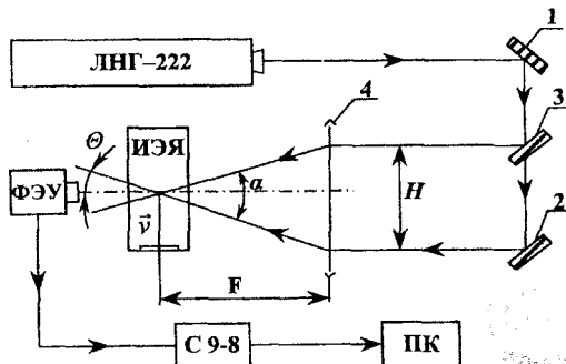
Рис. 1 – Схема лазерной доплеровской измерительной установки для определения электрофоретической скорости, эффективного диаметра и величины электрокинетического потенциала при электрофорезе
