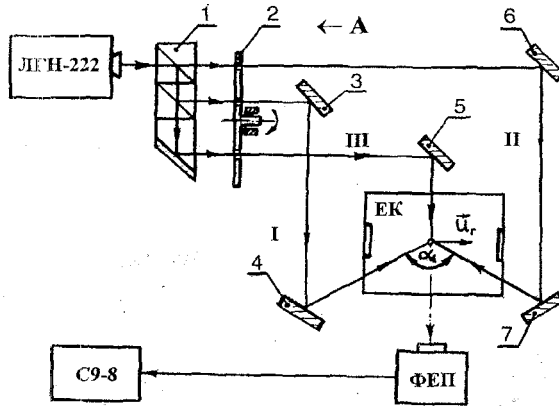
Оптическая схема лазерного доплерівського інтерферометра для вимірювання швидкості, дзета-потенціалу і ефективного діаметра частинок домішок
