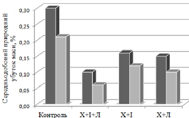
Рис. 3. Середньодобовий природний убуток маси під час зберігання плодів кабачка: ■ – Таміно; □ – Кавалі
