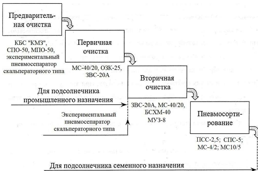
Схема технологическая послеуборочной обработки семян подсолнечника
