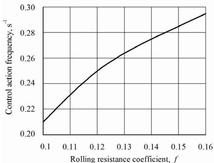
Рисунок 2 – Залежність бажаної частоти повороту керованих коліс агрегатуючого трактора комбінованого удобрювально-посівного машинно-тракторного агрегату від умов його руху (коефіцієнта опору коченню f )
