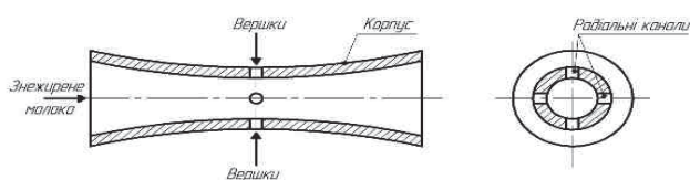
Рис. Схема струминного гомогенізатора молока з роздільним подаванням жирової фази
