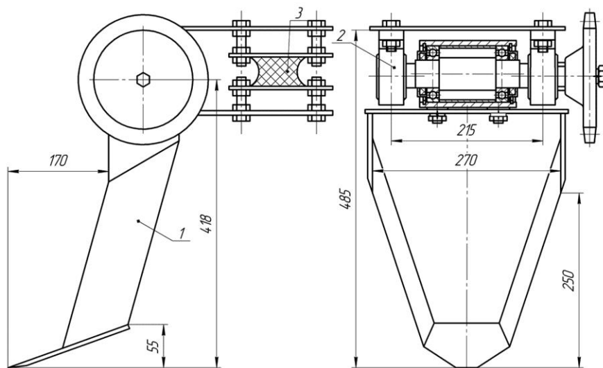
Рис. 2. Конструктивна схема дослідного зразка копача столових коренеплідів: 1 – корпус; 2 – ексцентриковий механізм; 3 – пружний елемент.
