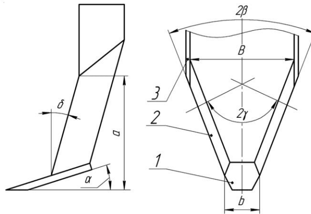
Рис. 1. Розрахункова схема V-подібного знаряддя: 1 – леміш; 2 – боковий стояк; 3 – несучий стояк
