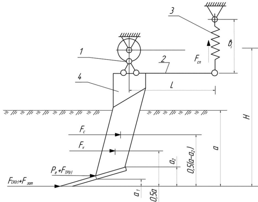
Рис. 3. Схема діючих сил у повздовжньо вертикальній площині:
