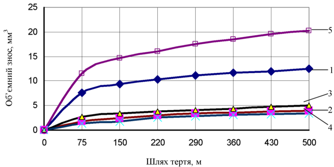
Рис.1-Залежність об'ємного зносу матеріалів від шляху відносного переміщення зразків в середовищі біопалива:
