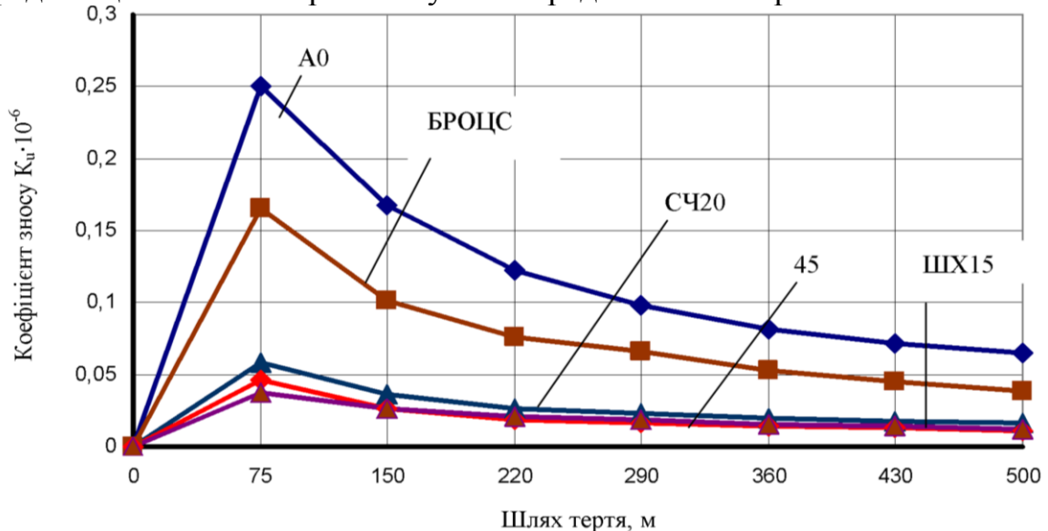
Рис.3. Зміна коефіцієнтів зносу різних матеріалів в середовищі біопалива при зношуванні.
