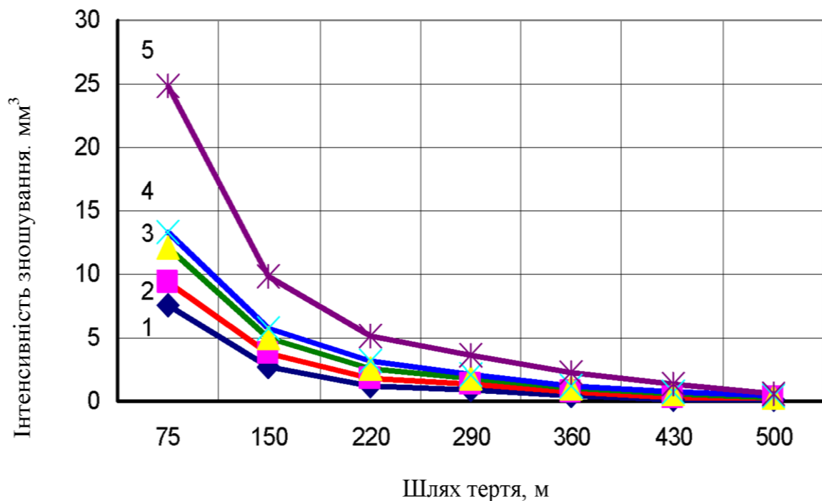
Рис.2- Інтенсивність зношування матеріалів в середовищі біопалива: 1- сталь 45, 2 – Сталь Шх15, 3 – сірий чавун Сч20, 4- бронза Бр ОЦС 5-5-5, 5 – алюміній А0.
