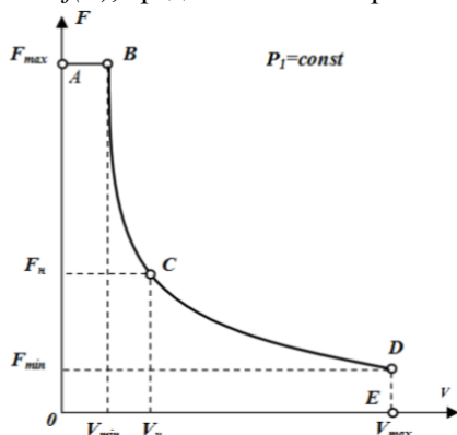
Рис. 1 – Предельная тяговая характеристика электромоторблока
