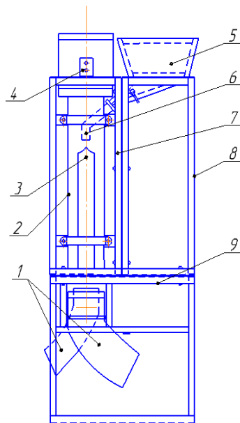
Рис.1. Схема пневмогравітаційного сепаратора насіння: 1 – два розподільника; 2 – аспіраційний канал; 3 – подільник; 4 – вентилятор; 5 – бункер; 6 – патрубок постачання; 7 – ліва частина рами; 8 – верхня частина рами; 9 – нижня частина рами
