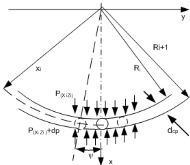
Рис. 1. Схема расположения материала на наклонной круговой поверхности.
