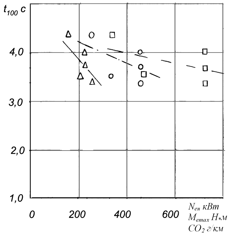
Рис. 2 Вплив показників двигуна на ХЧР ЛА: точки □ і лінія - - - для максимального крутного моменту, точки o і лінія - - - - - для номінальної потужності, точки Δ й лінія - - - - - для питомого викиду \text{CO}_2 .
