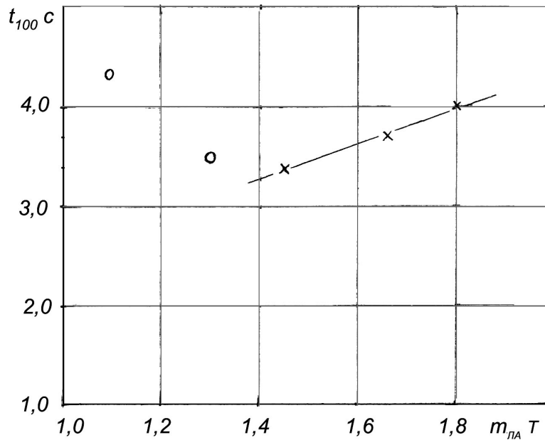
Рис. 1 Вплив маси ЛА на ХЧР (точки x для моделей Esprit, Elite і Eterne)
