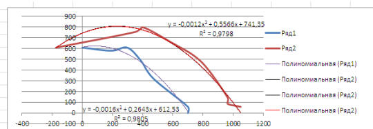
Рис. 7. Траектория полета частиц соломенной подстилки.
