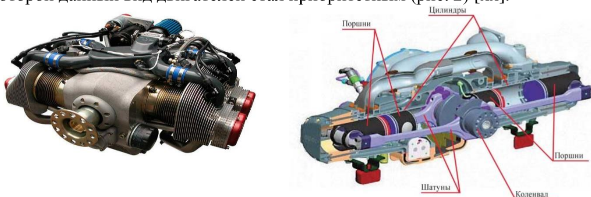
Рис. 2. Оппозитный двигатель Subaru
