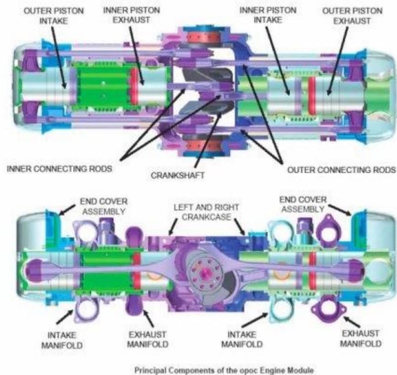
Рис. 4. Схема двигателя ОРОС
