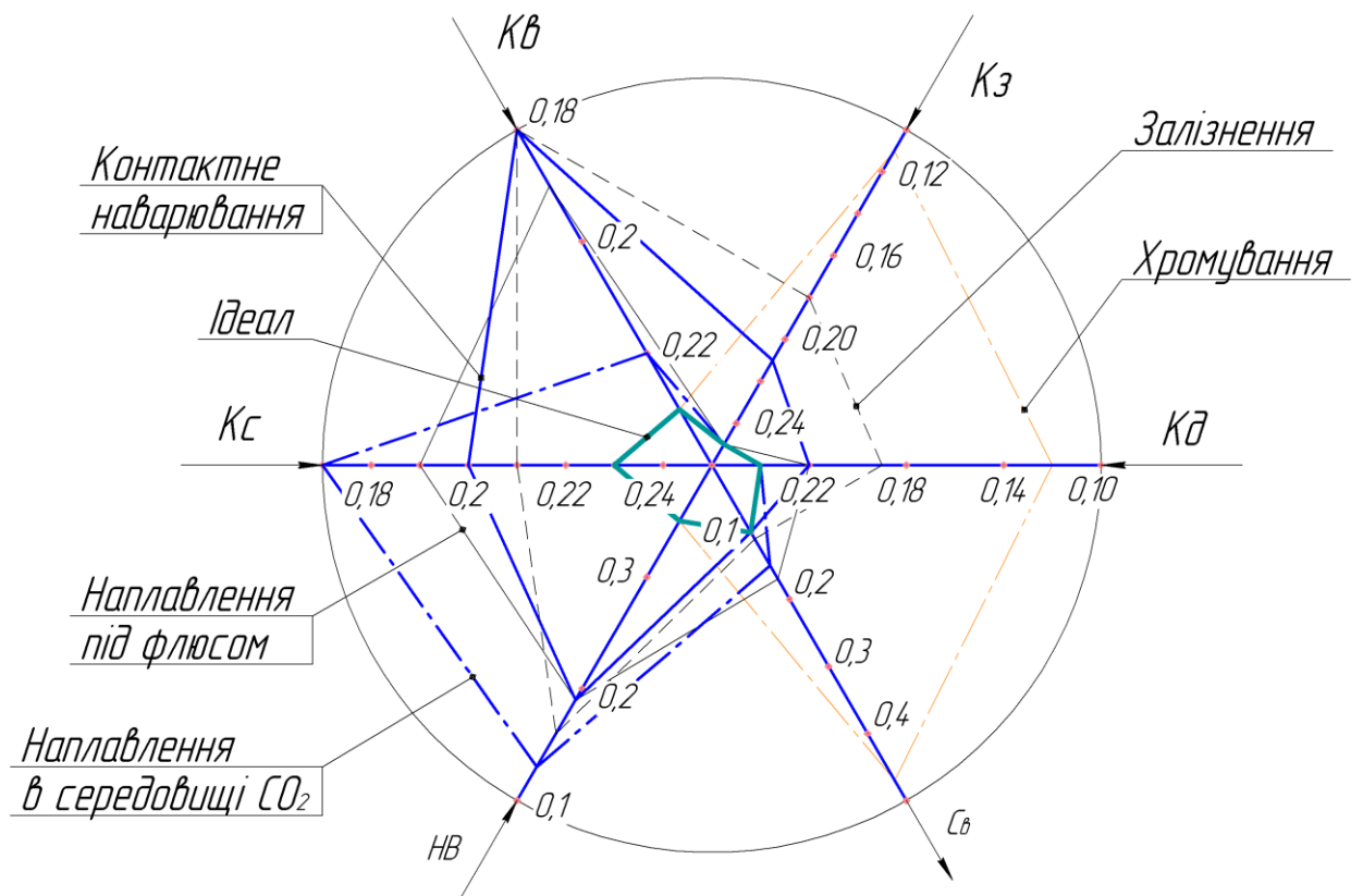
Рисунок 1 – Багатокритеріальна оцінка за відстанню до цілі
