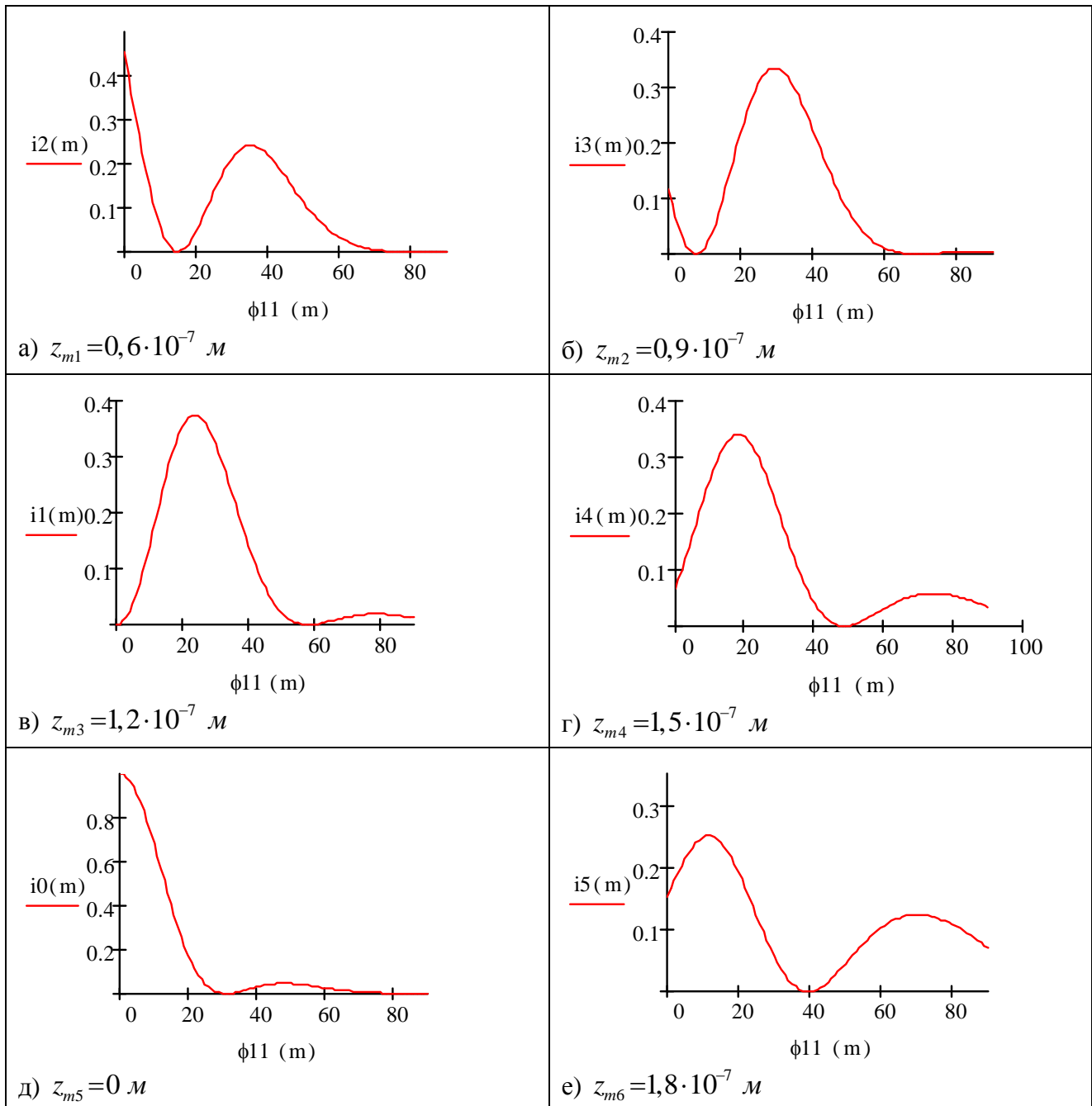
Рис. 2. Графіки залежності інтенсивності дифракційної хвилі від кута дифракції для різних значень амплітуди z_m модуляції рельєфу гармонічної ґратки.
