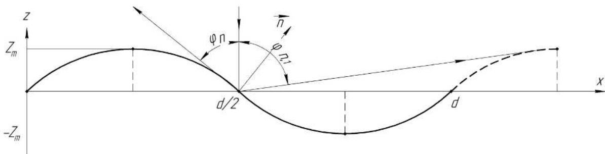
Рис. 1. Обмеження кутів дифракції при відбитті від гармонічної ґратки
