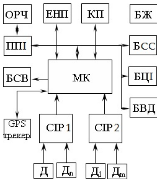
Рисунок 1 – Структурна схема побудови САУ опромінення рослин у теплиці
