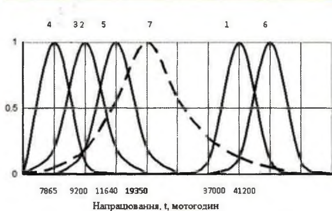
Рис. 2 – Середній ресурс паливної системи дизельного двигуна (7), який працює на МЕРО: 1 – ресурс паливного бака, 2 – ресурс помпи, 3 – ресурс фільтра, 4 – ресурс ПНВТ, 5 – ресурс форсунок, 6 – ресурс трубопроводів
