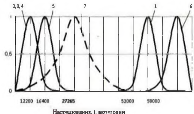
Рис. 1 – Середній ресурс паливної системи дизельного двигуна (7), який працює на ДП: 1 – ресурс паливного бака, 2 – ресурс помпи, 3 – ресурс фільтра, 4 – ресурс ПНВТ, 5 – ресурс форсунок, 6 – ресурс трубопроводів
