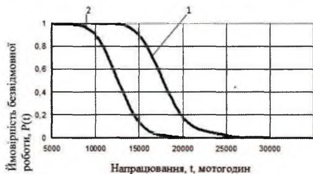
Рис. 3 – Ймовірність безвідмовної роботи паливних систем дизелів, які працюють на 1 – ДП, 2 – МЕРО
