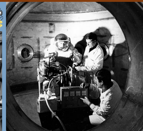
Відпрацювання режимів зварювання універсального ручного інструмента у відділі космічних технологій ІЕЗ імені Є. О. Патона
