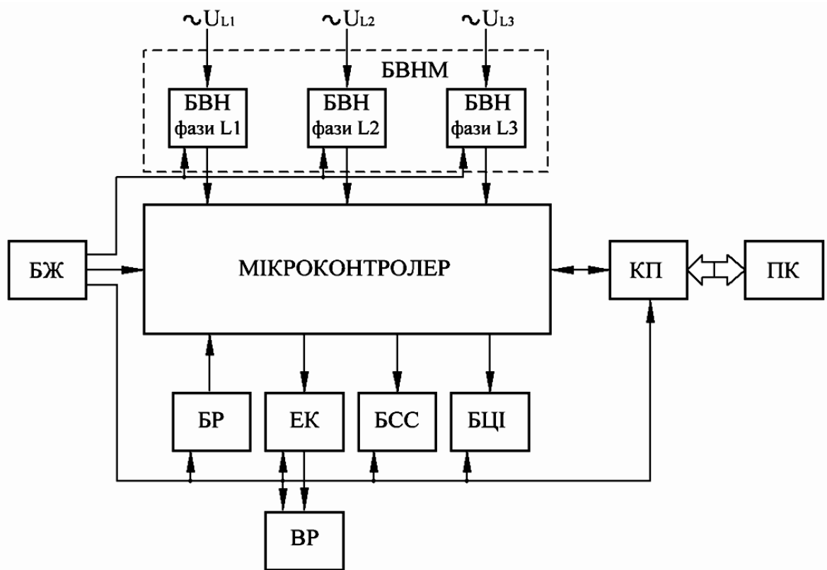
Рисунок 1. Пристрій захисту асинхронних двигунів від аномальної напруги мережі
