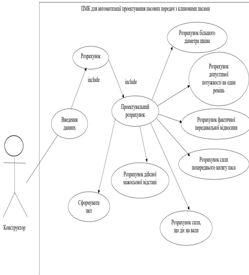
Рис. 1. Діаграма прецедентів ПЗ автоматизації проектування КПП
