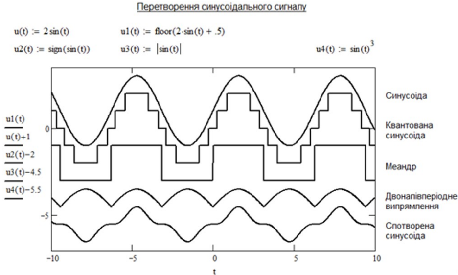
Рис. 2. Синусоїдальний сигнал і його перетворення
