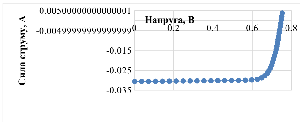
Рис. 1. Вольт-амперна характеристика фотоперетворювача CdS/CdTe
