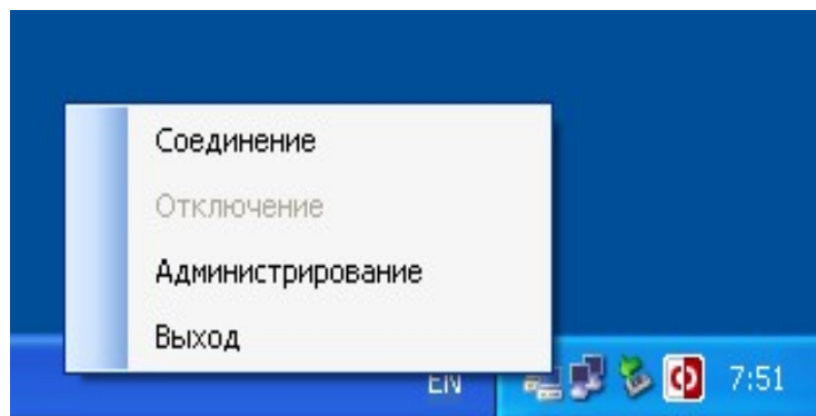
Рис. 1. Windows-клієнт
