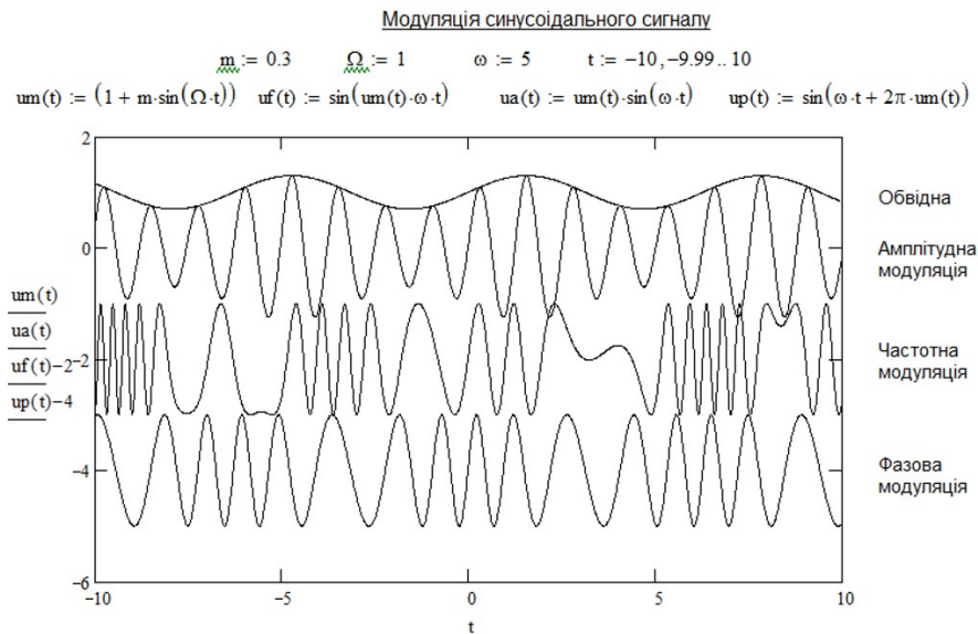
Рис. 3. Види модуляції синусоїдального сигналу
