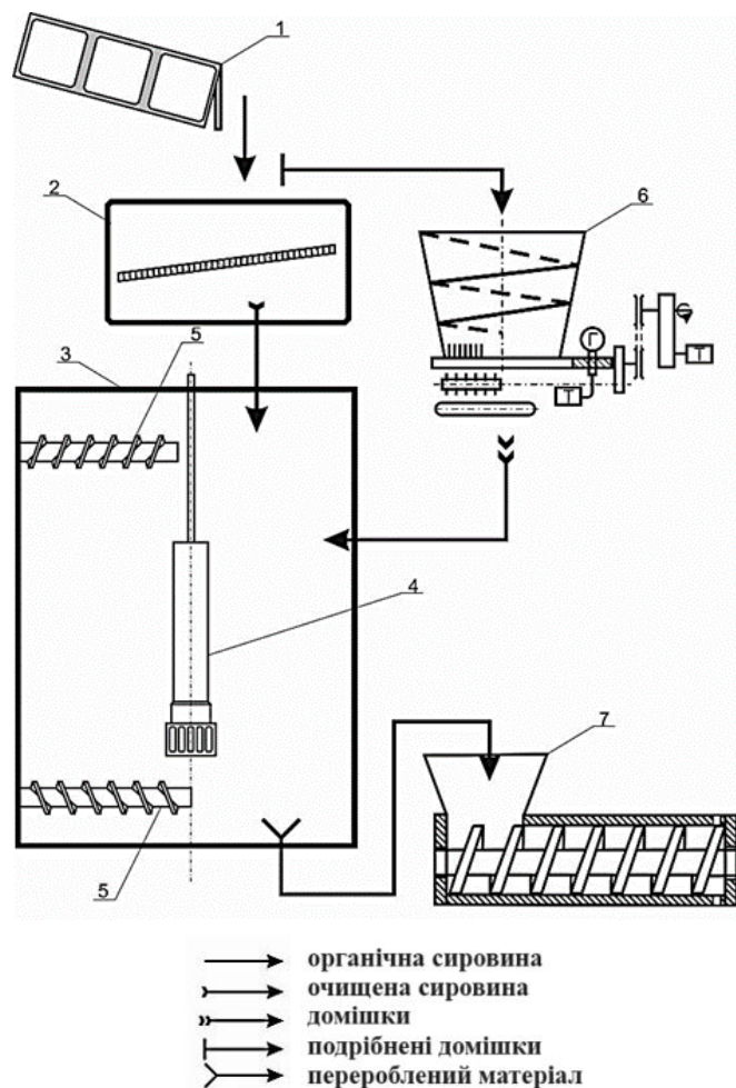
Рис. 2. Загальна схема технологічного процесу функціонування біогазової установки: 1 – бункер з сировиною, 2 – вібросито, 3 – біореактор, 4 – диспергатор, 5 – змішувальний шнек, 6 – подрібнювач, 7 – гвинтовий прес
