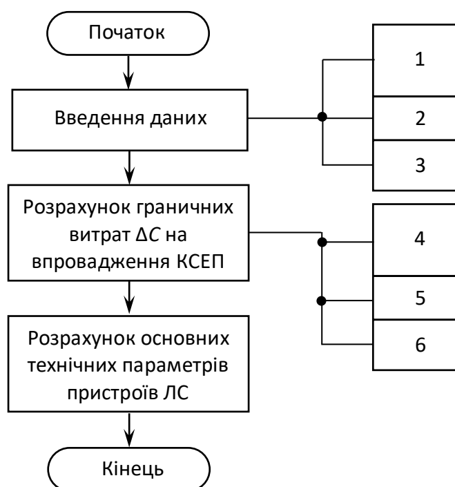
Рисунок 3. Структурна схема алгоритму визначення \Delta C та основних технічних параметрів пристроїв локальної системи електропостачання, куди входять вхідні компоненти програми:
