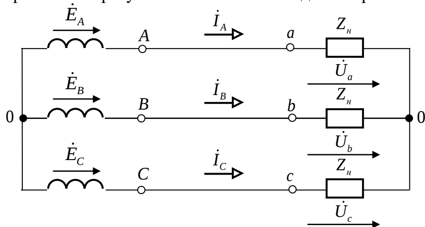
Рис. 1. Розрахункова схема трифазного кола «зірка – зірка» зі статичним навантаженням у симетричному режимі
