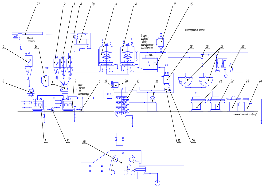
Рис. 1. Апаратурно-технологічна схема виготовлення майонезу:
