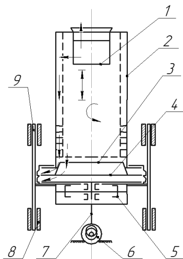
Рис. 1. Схема віброцентрифуги [14]:
