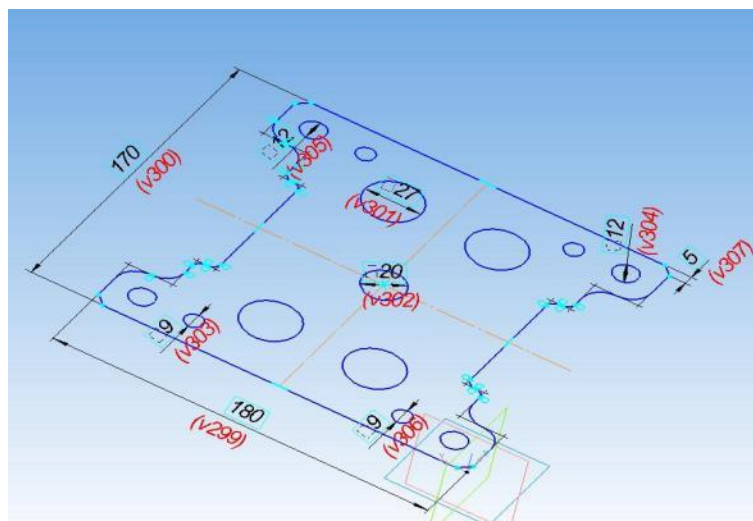
Рисунок 4. Ескіз деталі
