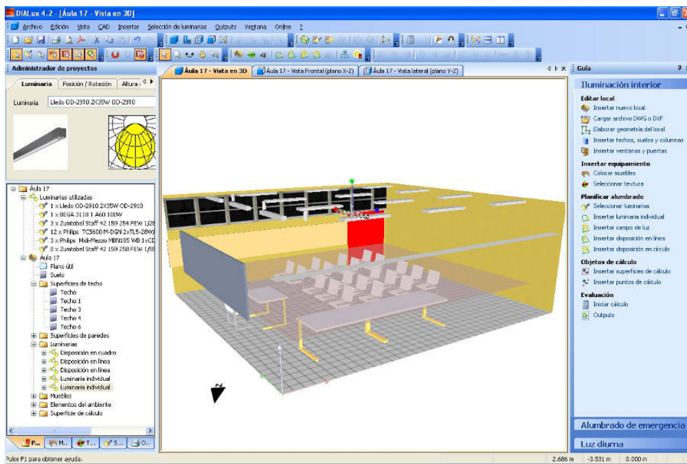
Рис. 3. Інтерфейс Dialux
