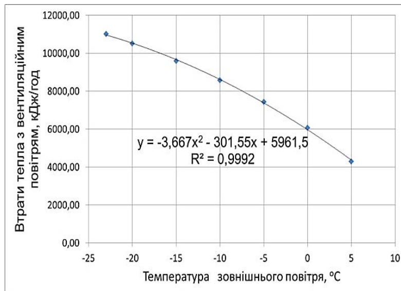
Рисунок 3. Залежність втрат теплової енергії з вентиляційним повітрям природної вентиляції тваринницького приміщення від температури зовнішнього повітря при tt_{\text{в}} = 10^{\circ}\text{C}
