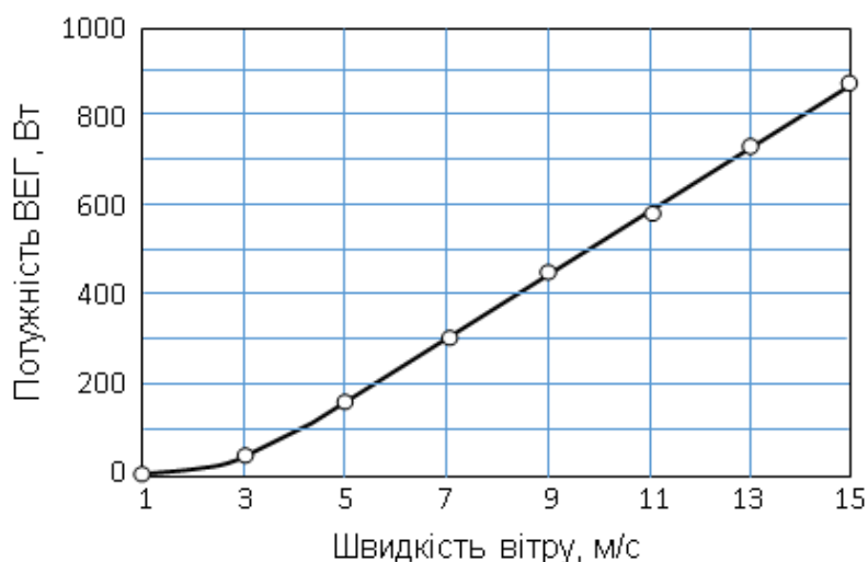
Рисунок 4. Залежність потужності ВЕР від швидкості вітру при струмі навантаження 25 А
