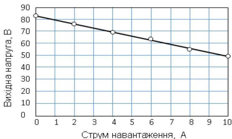
Рисунок 3. Зовнішня характеристика ВЕР
