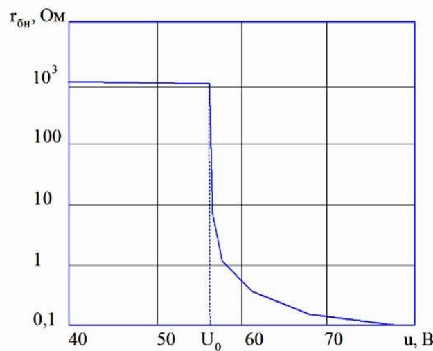
Рисунок 6. Опір баластного навантаження r_{\text{бн}}
