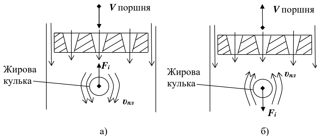
Рисунок 1. Схема виникнення сил інерції при імпульсній гомогенізації при русі поршня-ударника: а) вниз; б) ввєрх.
