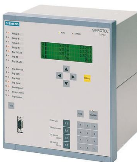
Рисунок. 3. Вид з лицьової частини мікропроцесорного терміналу релейного захисту SIEMENS SIPROTEC
