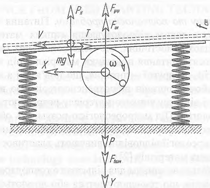
Рис. 2. Схема дебалансного вібраційного дозатора.
