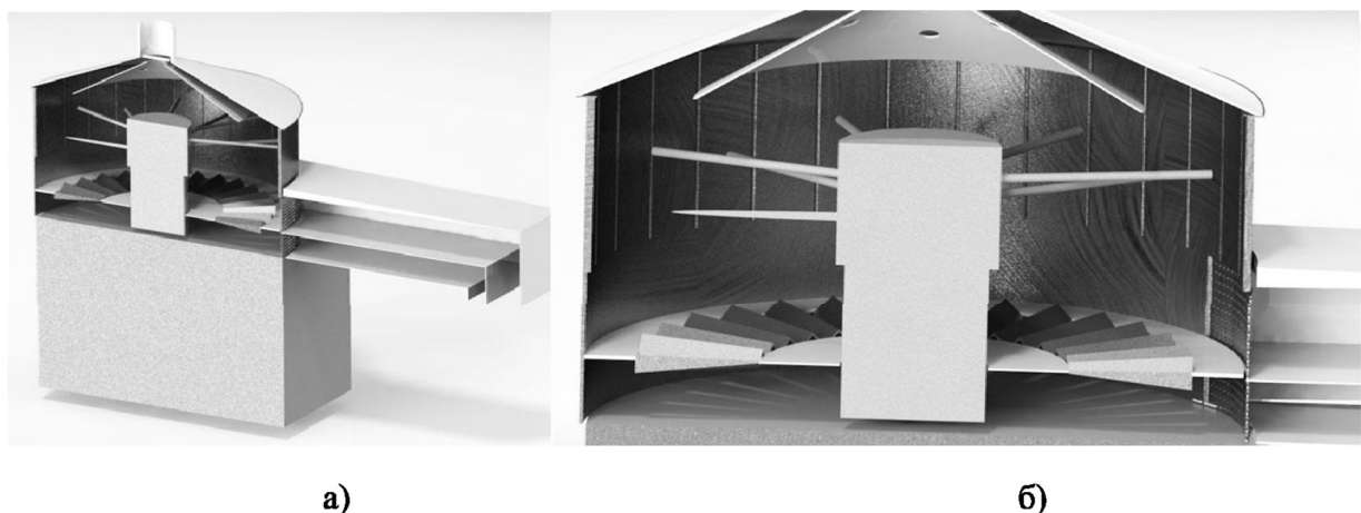
Рис. 2. 3-D модель пальцевої дробарки з вертикальним ротором: а) загальний вигляд; б) робоча камера
