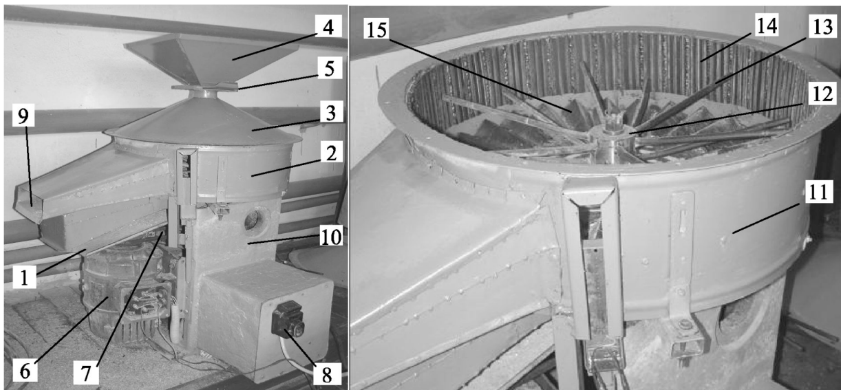
Рис. 1. Фото загального вигляду і робочої камери дробарки:
