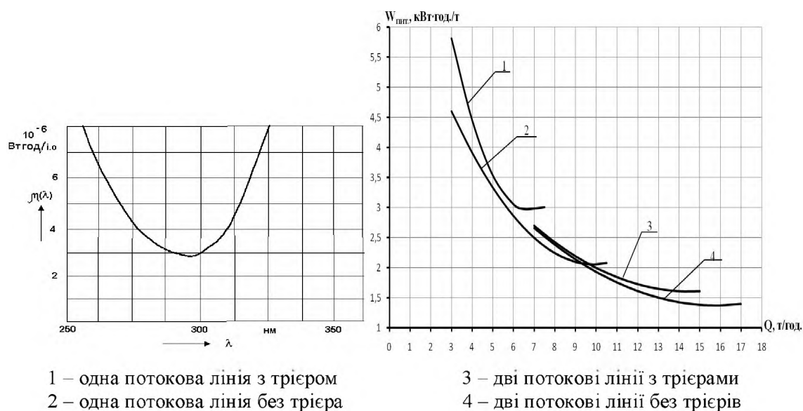
Рис. 1. Залежності питомих витрат електроенергії в функції продуктивності поточкових ліній при оптимальних значеннях вологості та засміченості.
