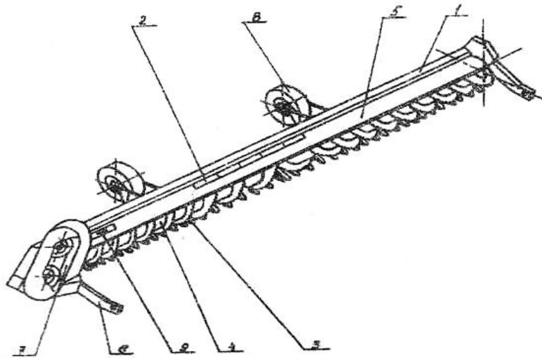
Рис. 3 - Схема шнекового апарату різання АРШ-4,0:
