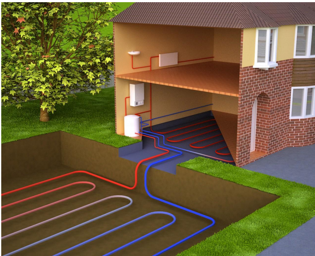
Рис. 2. Горизонтальний теплообмінник
