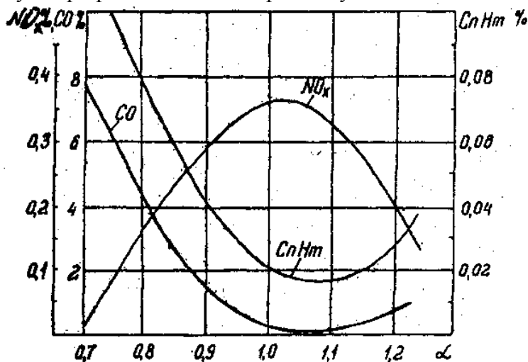
Рисунок 1 – Характеристика токсичності двигуна ЗІЛ-130
