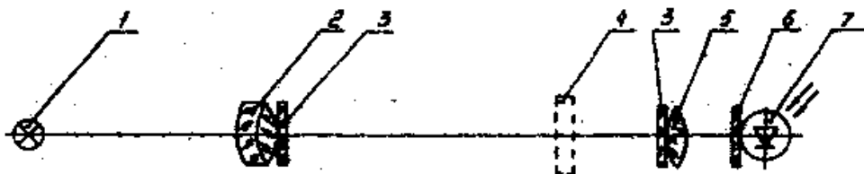
1 – лампа; 2 – об’єктив; 3 – скло; 4 – світлофільтр перевірочний; 5 – лінза; 6 – світлофільтр; 7 – фотодіод.
