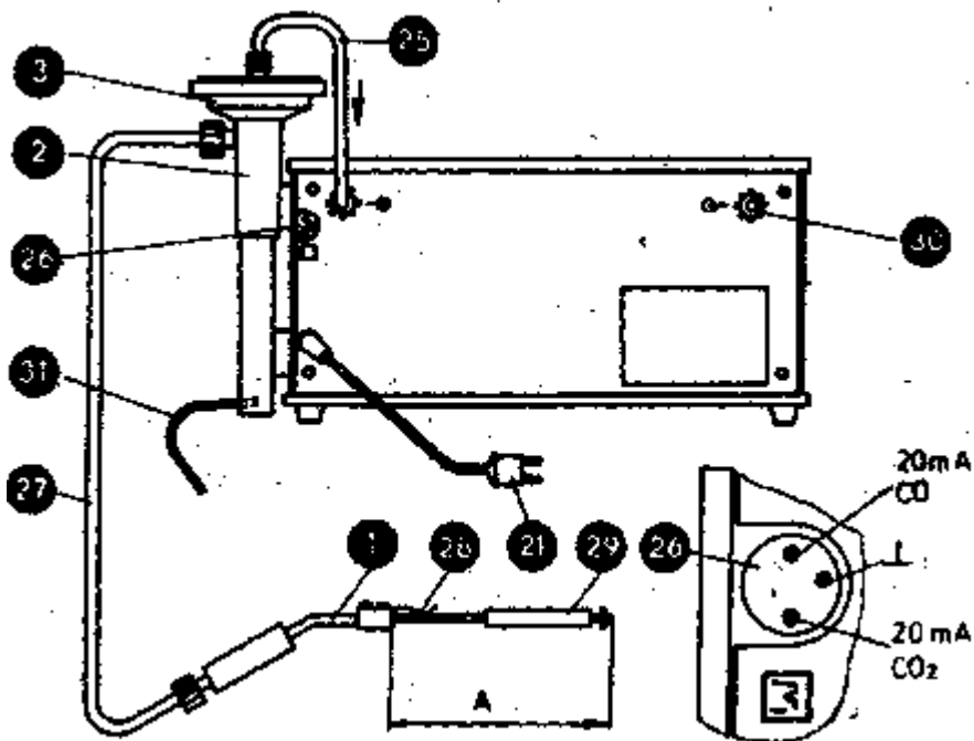
Рисунок 4 – Органи керування приладу (вид ззаду)
