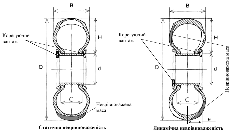
Рисунок 1 – Статична неврівноваженість
