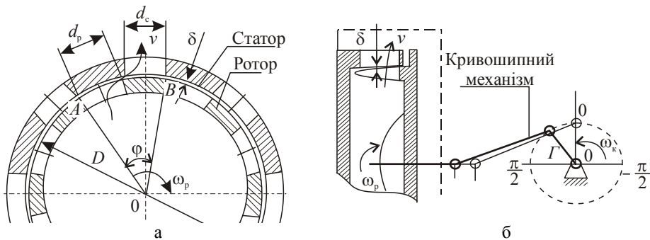
Рис. 1. Схема обертового і коливального рухів ротора ПА:
